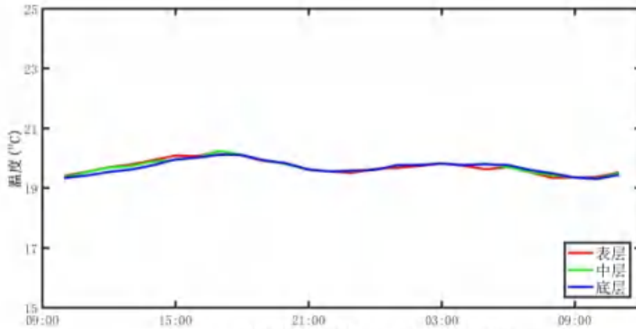
图 4.2-61 调查海域大潮 C12 站实测温度图
