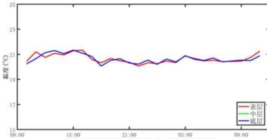
图 4.2-58 调查海域大潮 C9 站实测温度图
