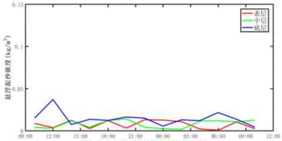
图 4.2-70 C6 站悬浮泥沙浓度曲线
