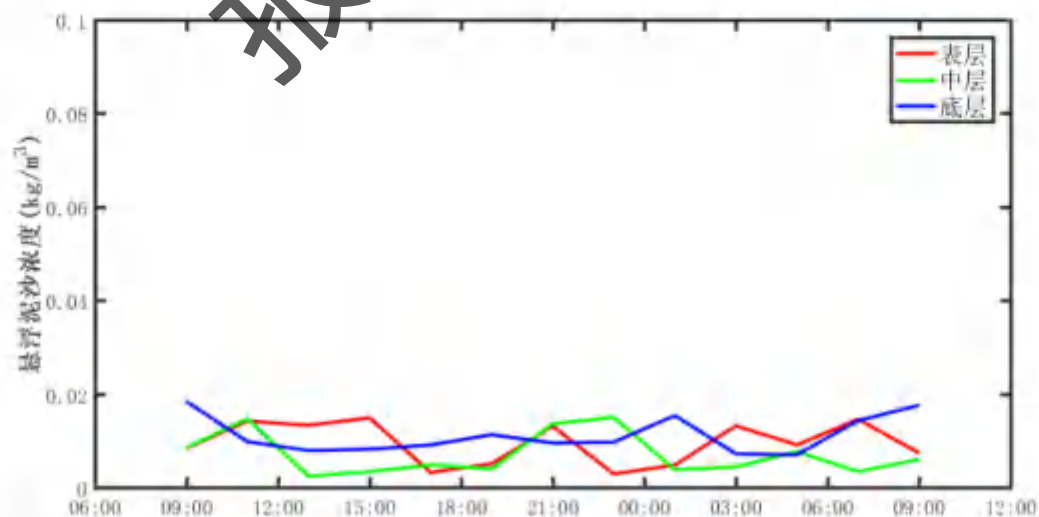
图 4.2-30C7 站悬浮泥沙浓度曲线
