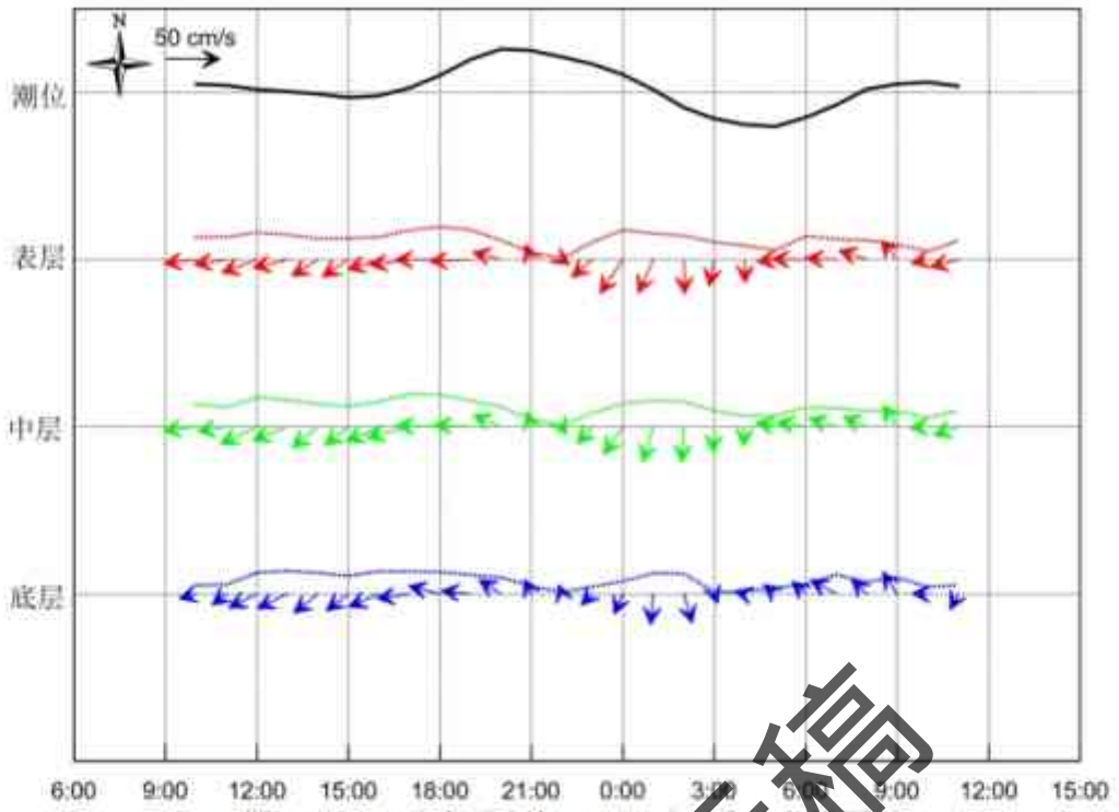
图 4.2-46 调查海域大潮 C12 站实测海流矢量图
