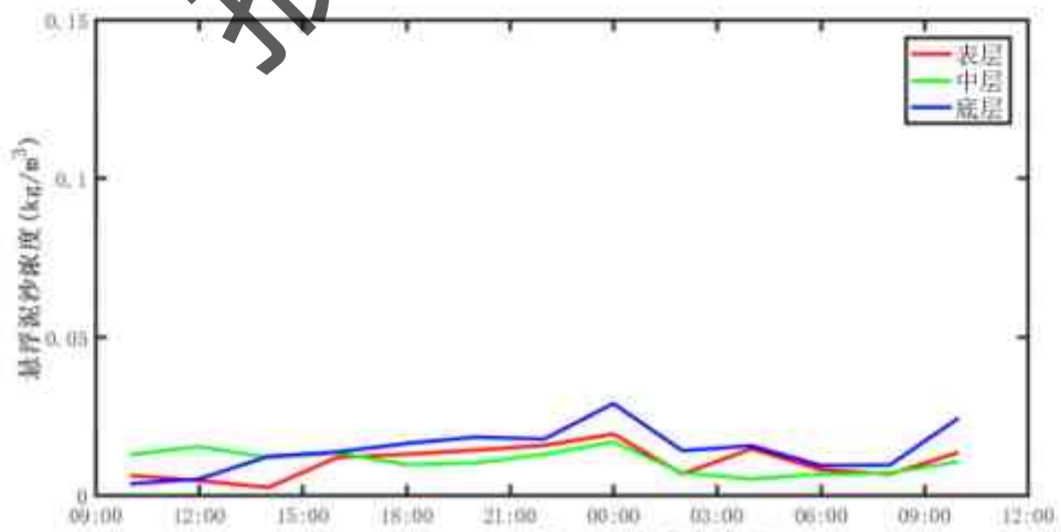
图4.2-75 C12站悬浮泥沙浓度曲线
