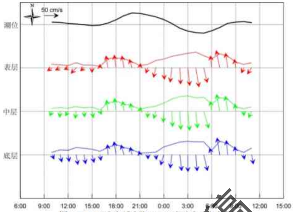
图 4.2-42 调查海域大潮 C8 站实测海流矢量图
