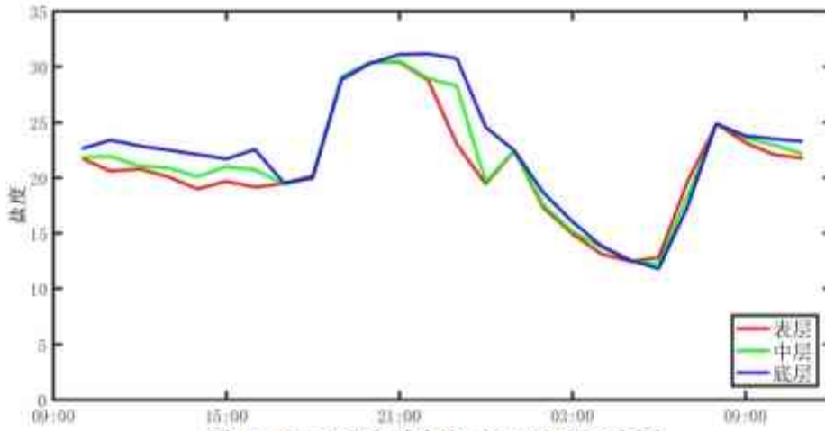
图 4.2-64 调查海域大潮 C8 站实测盐度图
