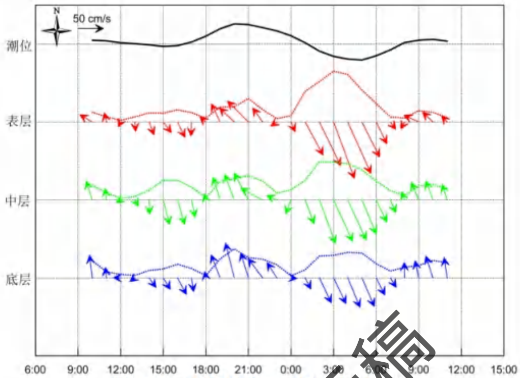
图 4.2-44 调查海域大潮 C10 站实测海流矢量图
