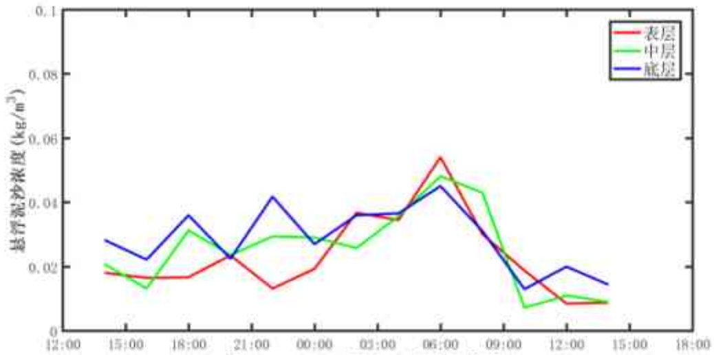
图 4.2-31C8 站悬浮泥沙浓度曲线
