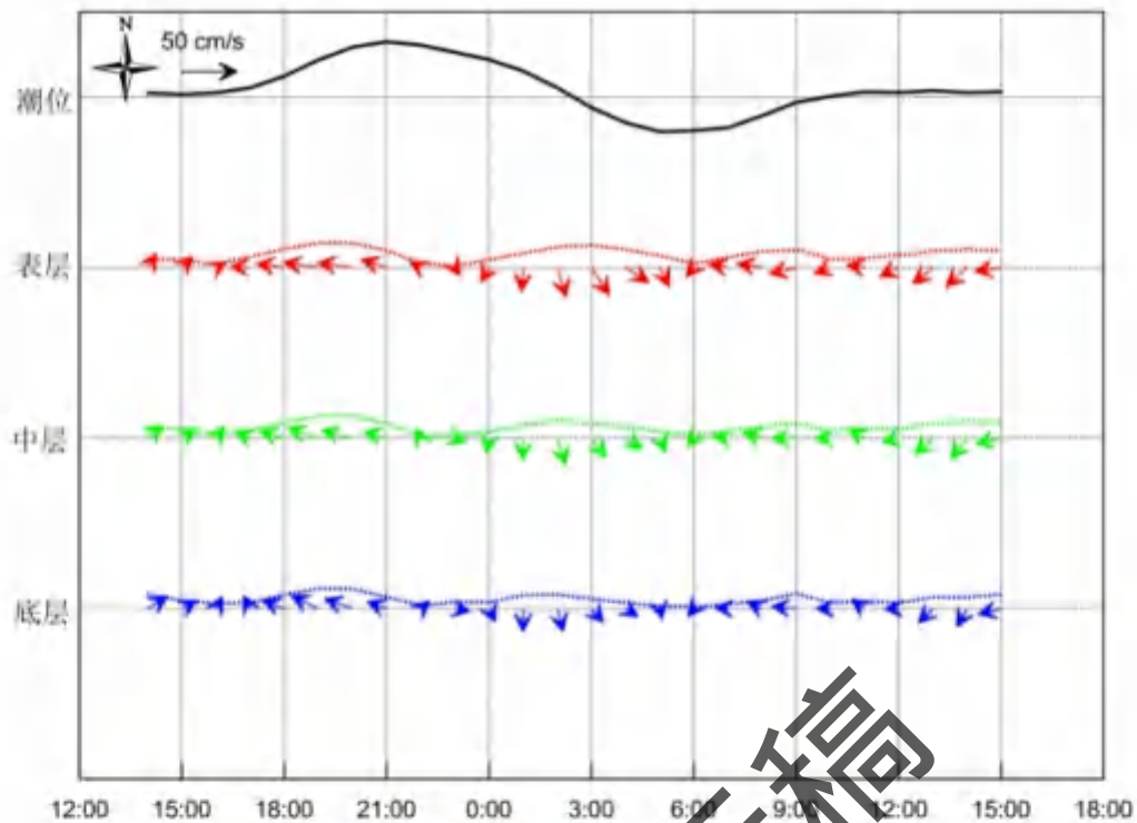
图 4.2-9 调查海域大潮 C12 站实测海流矢量图
