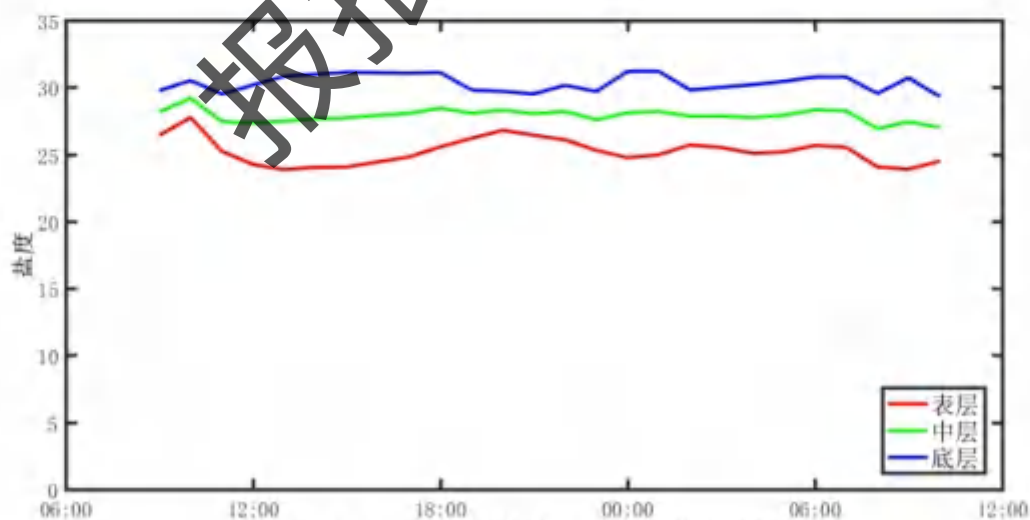
图 4.2-24 调查海域大潮 C7 站实测盐度图
