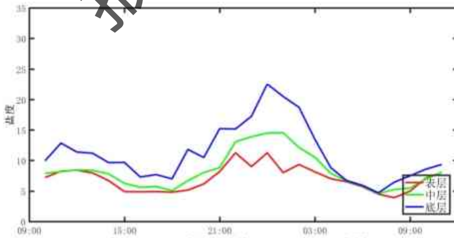
图 4.2-66 调查海域大潮 C10 站实测盐度图
