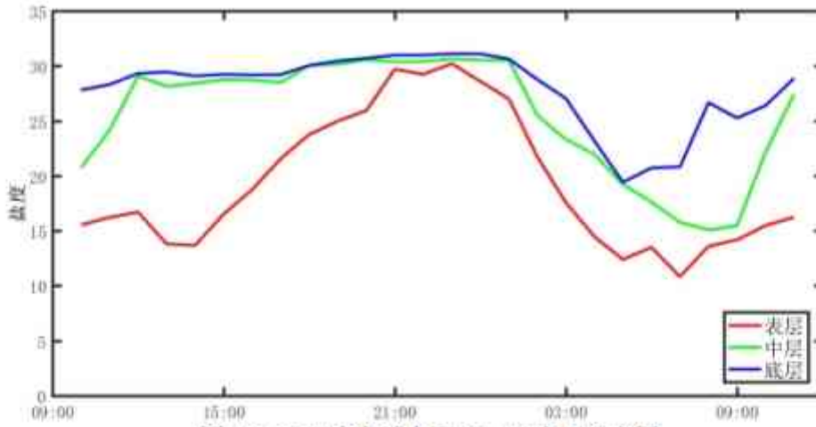
图 4.2-67 调查海域大潮 C11 站实测盐度图
