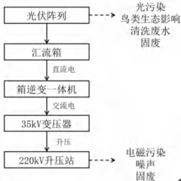
图 3.5-2 运营期工艺流程与产污环节
